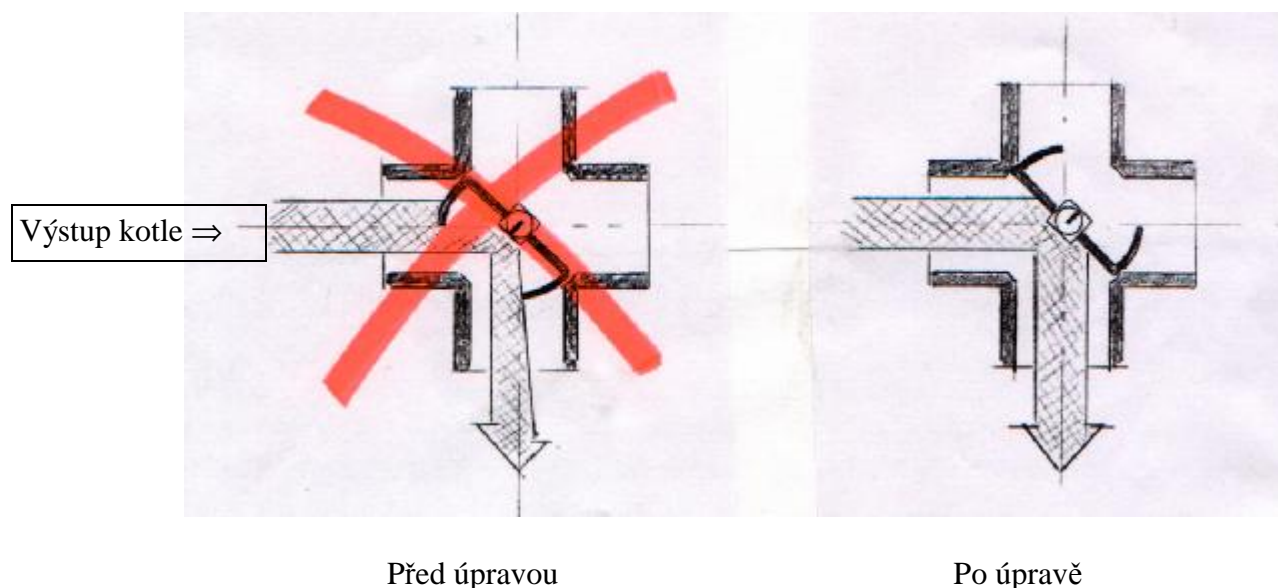
Obr. 6 Úprava čtyřcestného ventilu DUOMIX v systému se samotížným primárním okruhem (poloha rysky na hřídeli v poloze „ 0 „ = ZAVŘENO)
