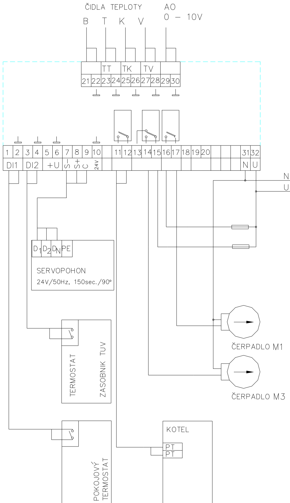
Obr. 9 Základní zapojení regulátoru EKVI DIN
