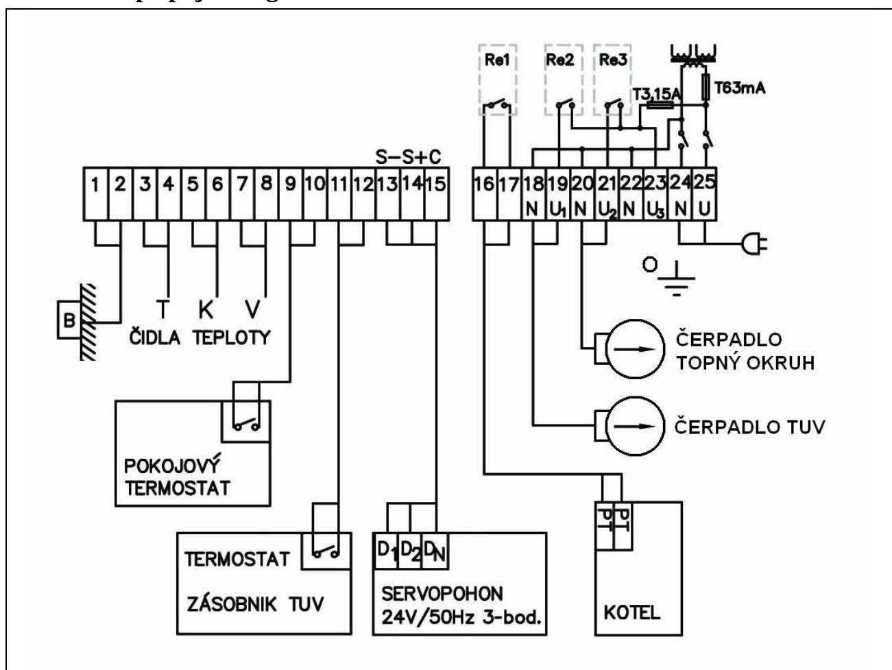
Obr. 18 Elektrické připojení regulátoru
