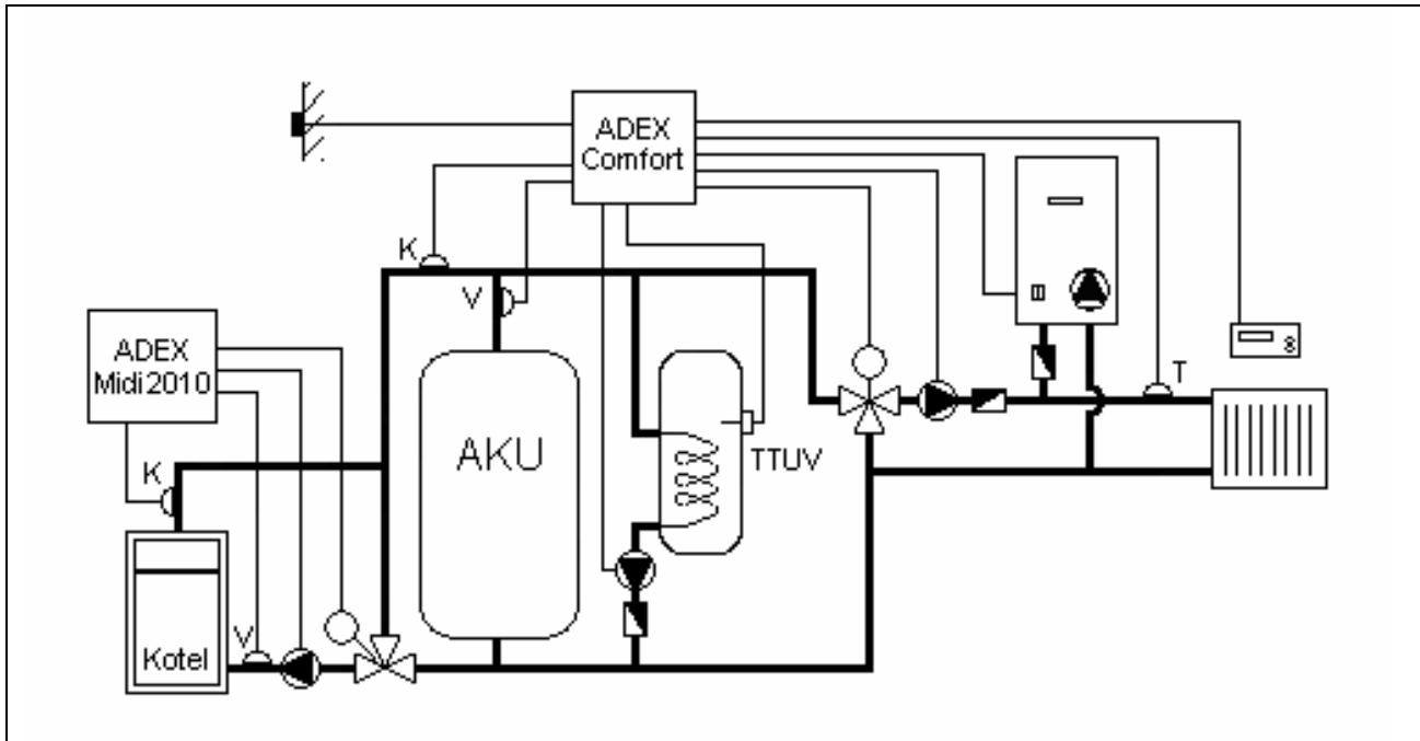
Obr. 15 Funkční schéma zapojení pro Systém 7
