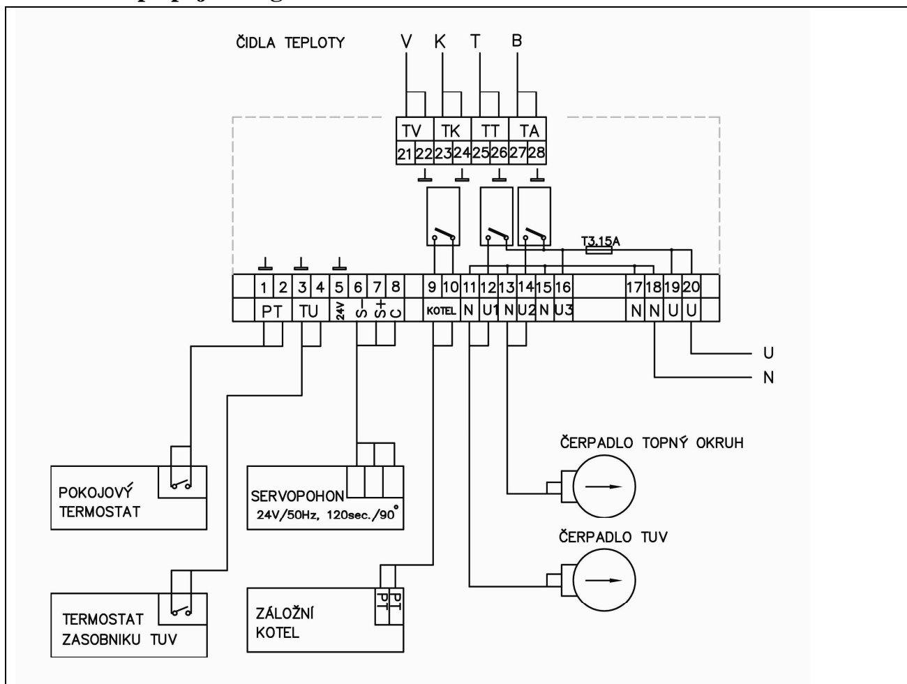
Obr. 16 Elektrické připojení regulátoru
