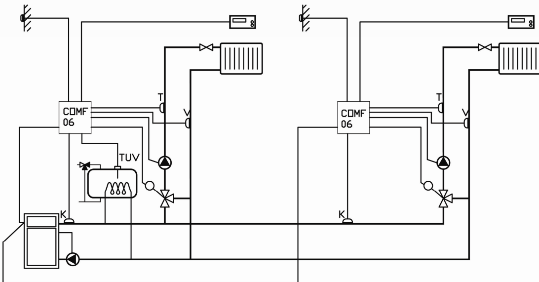
◀ Topný systém s kontrolou výstupní kotlové vody
